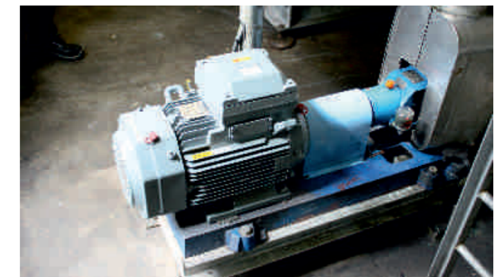
Baureihe CNH-B50-200, Förderdaten 60 m 3 /h, Medium Glykol/Wasser, Prozess Kühlsystem
